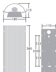
Настенный светильник Garbo Wall
