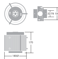
Потолочный светильник Garbo Ceiling
