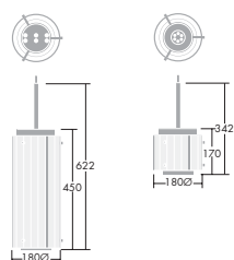
Подвесной светильник Garbo Pendant
